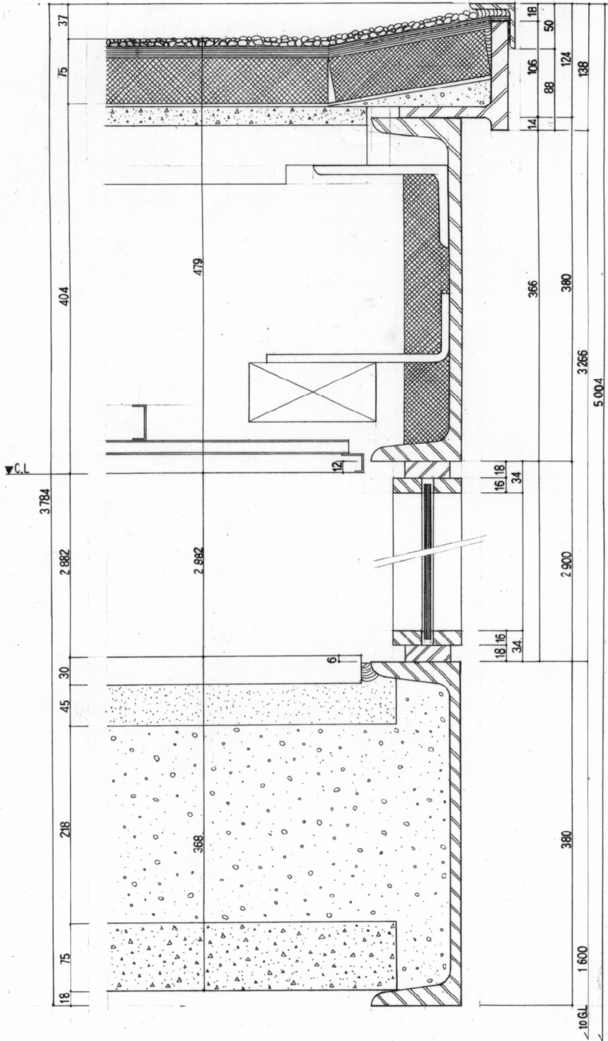
Farnsworth House 部分詳細図(4)
